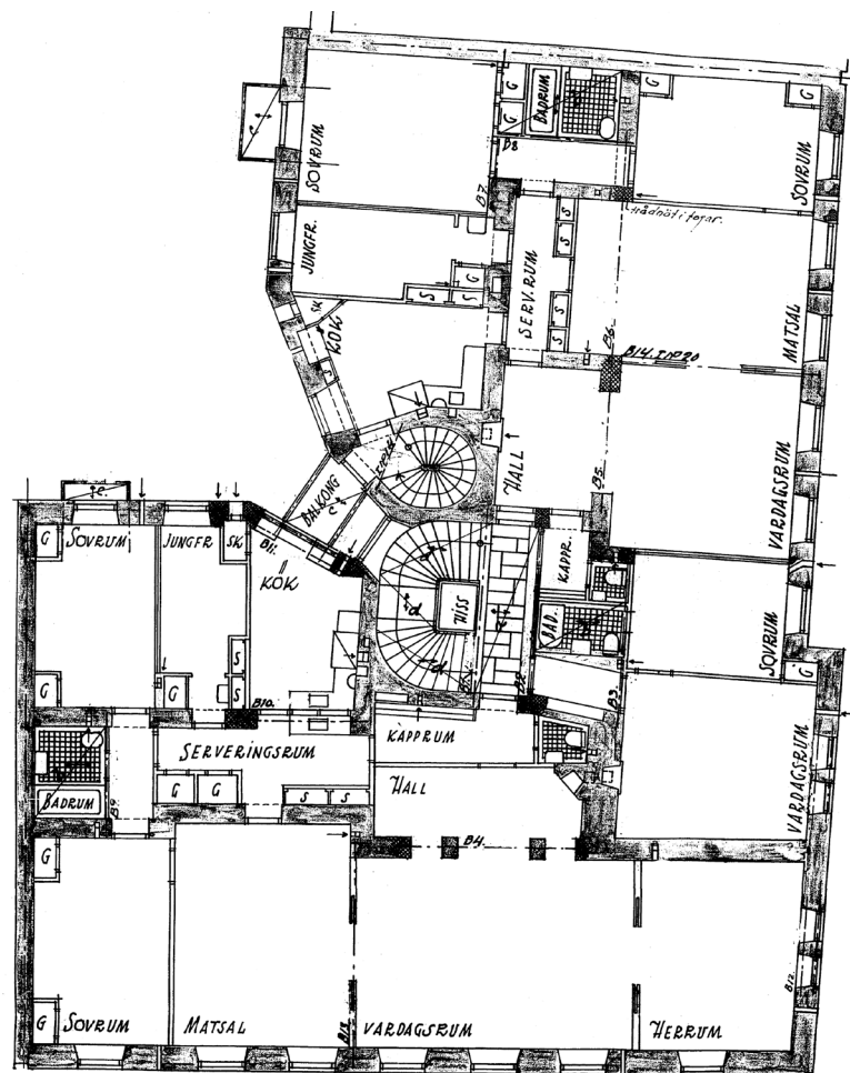
Ritning av plan 1 från 1928, signerad arkitekt Hugo Jahnke.
